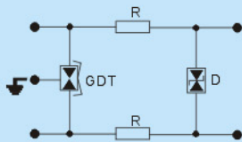
B180-T/MJ6 图解 GDT: 3极气体放电管 R: 电阻 D3: 3箱位二极管
